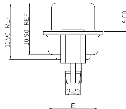
鉚合型
