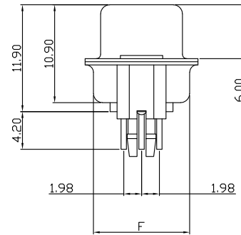
鉚合型
