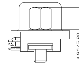
鉚合鎖螺絲型
