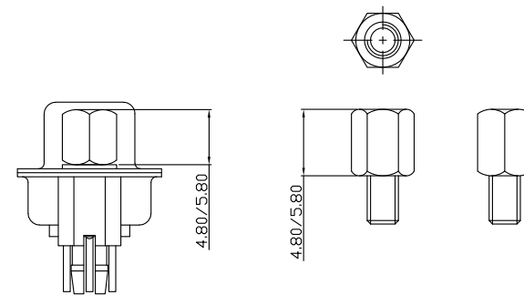
鉗合鎖螺絲型
