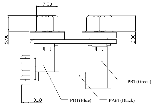
鉚合鎖螺絲型
