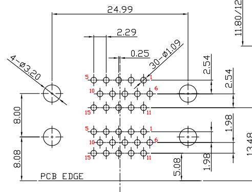
P.C.B. LAYOUT
