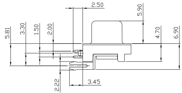
鉚合型
